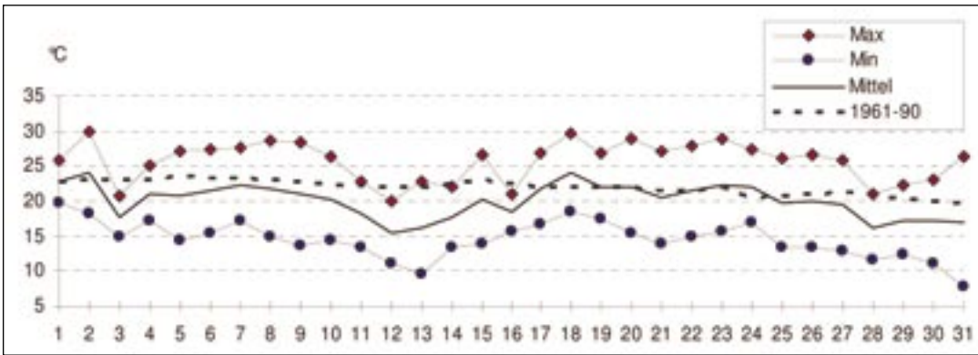
Die täglichen Temperaturen in Bozen zeigen, dass es oft zu kühl war. Nur zwischen dem 17. und 27. lagen die Werte nahe der Norm.
